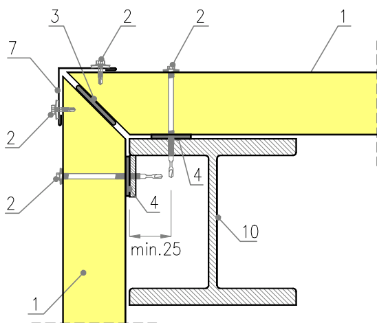
Horizontālās uzstādīšanas I veids
