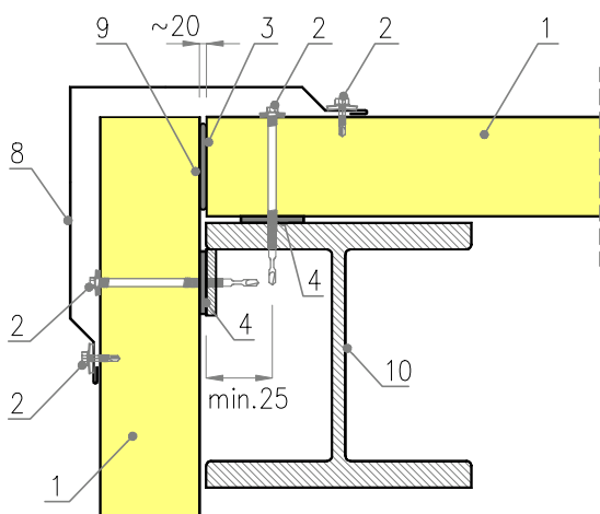
Horizontālās uzstādīšanas II veids:
