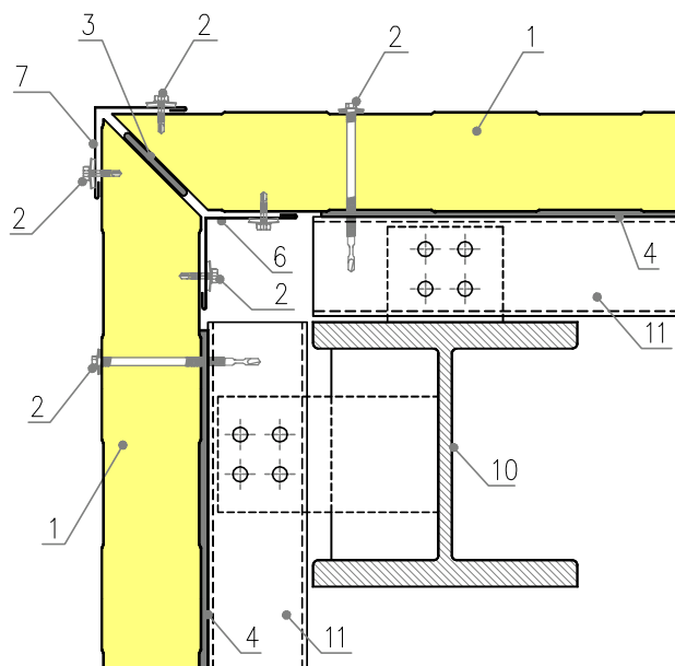
Vertikālās uzstādīšanas II veids:
