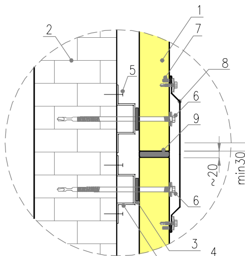
HORIZONTĀLĀ SISTĒMA – PANEĻU SAVIENOJUMS
