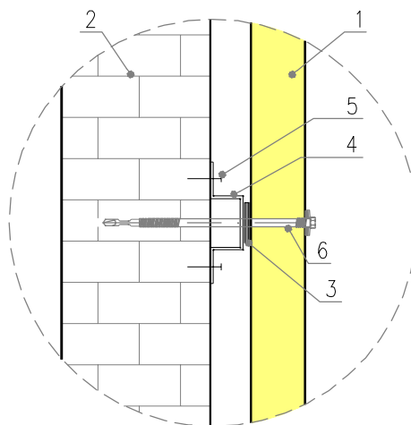
VERTIKĀLĀ SISTĒMA – STARPPOSMA ATBALSTS
